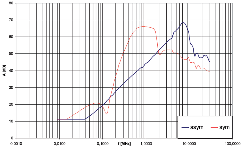
Dämpfungsverlauf CNW 101/16*
