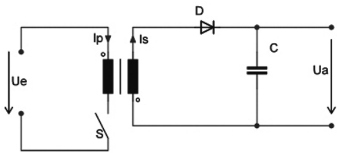
Schaltprinzip Sperrwandler
