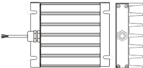
Bauform IP65
