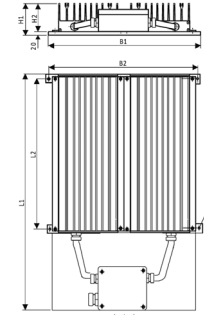
Maßbild, Bauform 1
