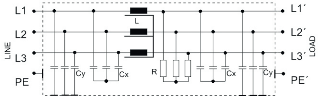
Schaltungsbeispiel
