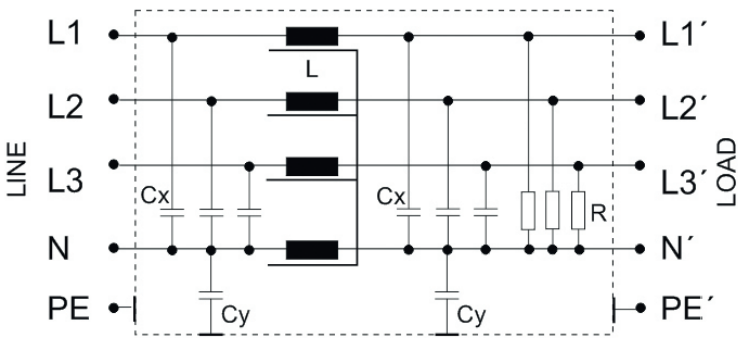
Schaltungsbeispiel
