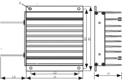
Bauform IP20
