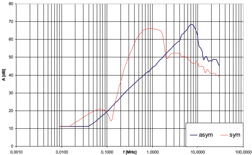
Dämpfungsverlauf CNW 101/16*
