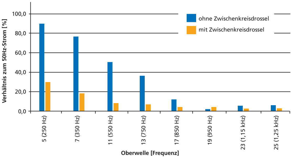
Vergleich der Oberwellen
