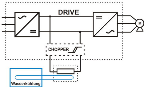
Schaltungsbeispiel
