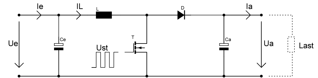
Schaltungsprinzip Hochsetzstellerdrossel
