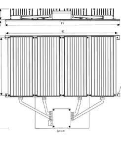
Maßbild, Bauform 3
