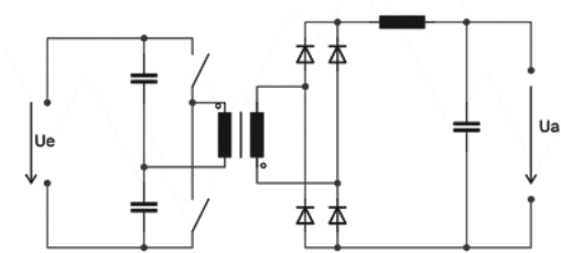
Schaltprinzip Halbbrücken-Gegentaktwandler
