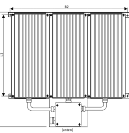
Bauform IP65
