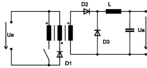
Schaltprinzip Durchflusswandler
