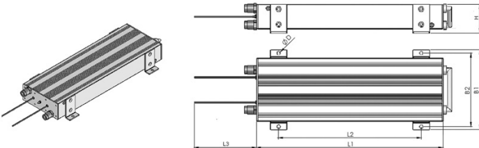
Maßbild, Bauform 1
