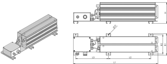
Maßbild, Bauform 2
