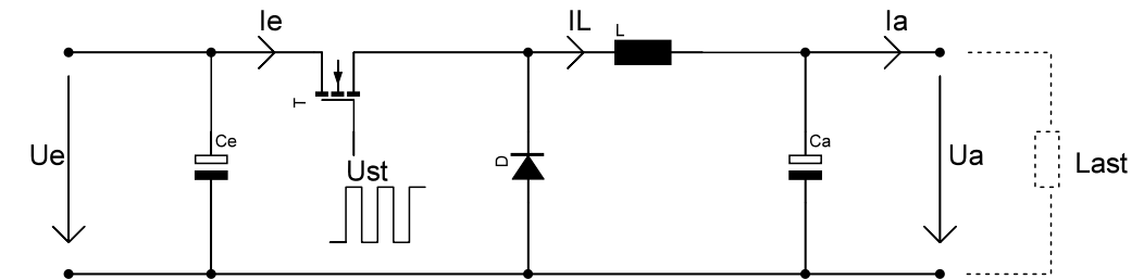
Schaltungsprinzip Tiefsetzstellerdrossel
