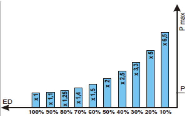
Belastungsdiagramm
