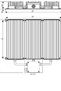
Maßbild, Bauform 2
