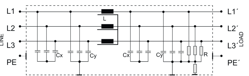
Schaltungsbeispiel
